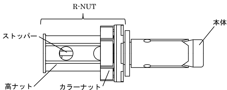
図 2. 製品概要図
