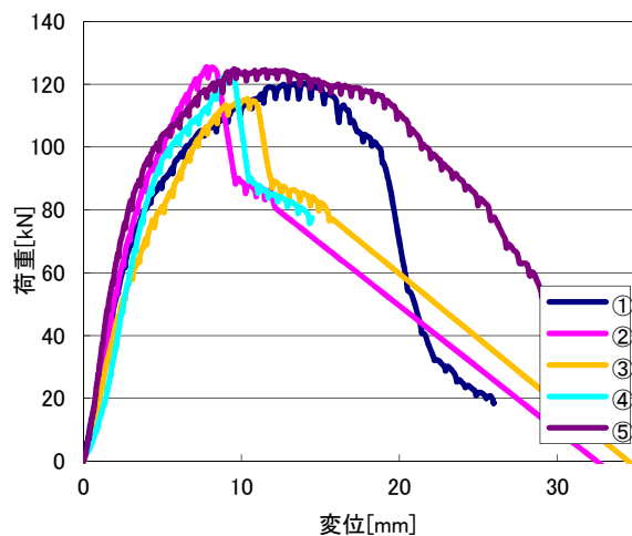
図1. 荷重変位曲線
